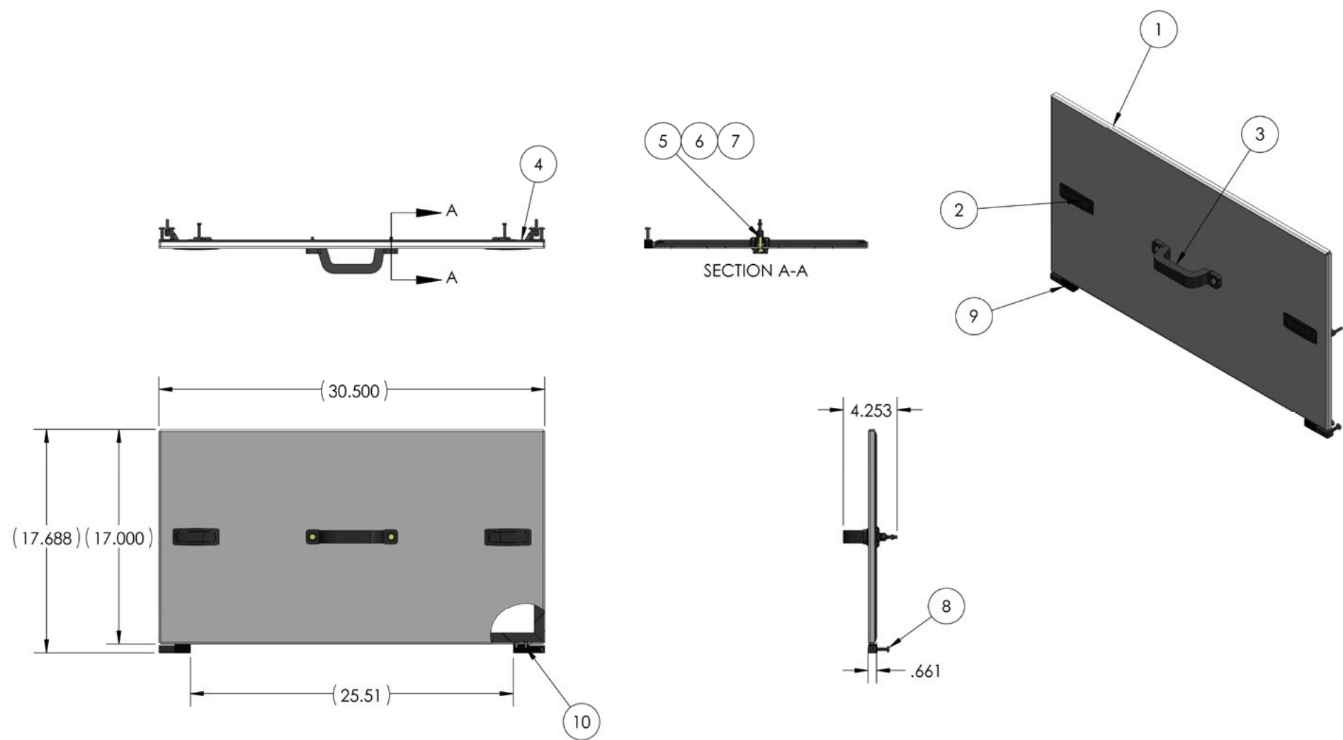
Hopper Side Door - Diagram 5
